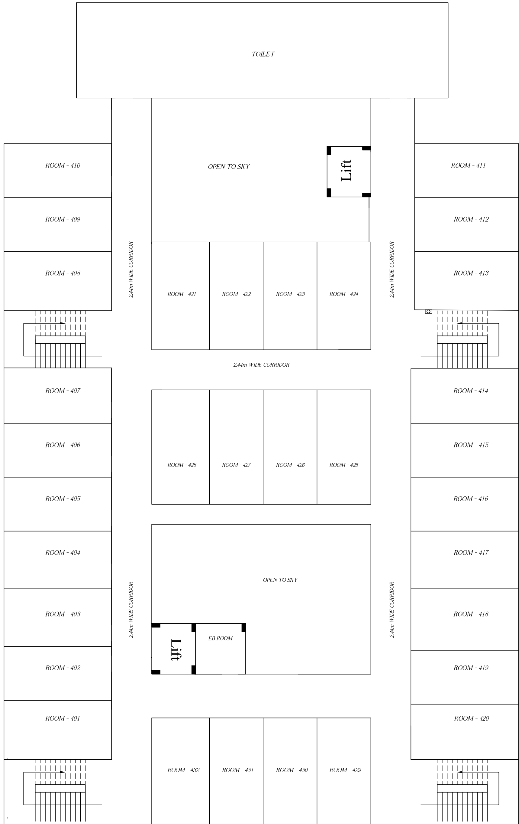
THIRD FLOOR PLAN OORI 'T BLOCK
