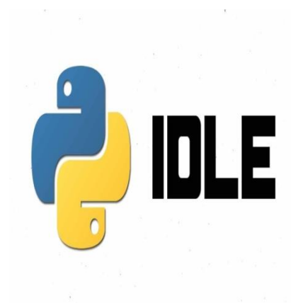
Python IDLE
